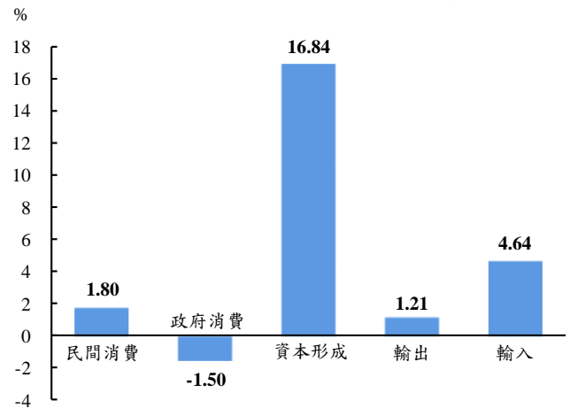
107Q3 GDP各項支出成長率
