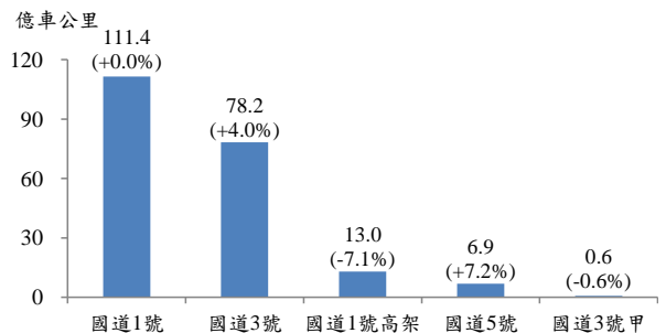
109年1-8月高速公路延車公里-國道別
